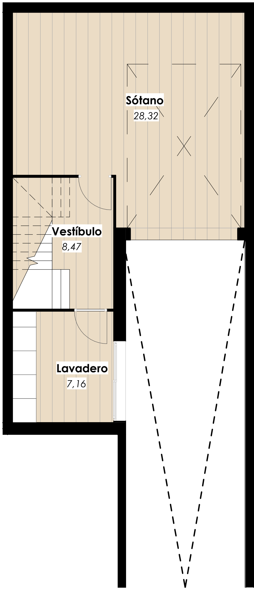
PLANTA GARAJE
